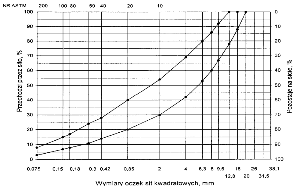
Rys. 2. Krzywe graniczne uziarnienia mieszanek mineralnych BA od 0 do 16 mm do warstwy wiążącej i wyrównawczej nawierzchni drogi o obciążeniu ruchem od KR2
